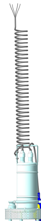
Рисунок Д.2 - Общий вид спирального кабеля на электронасосе с автоматизацией.
