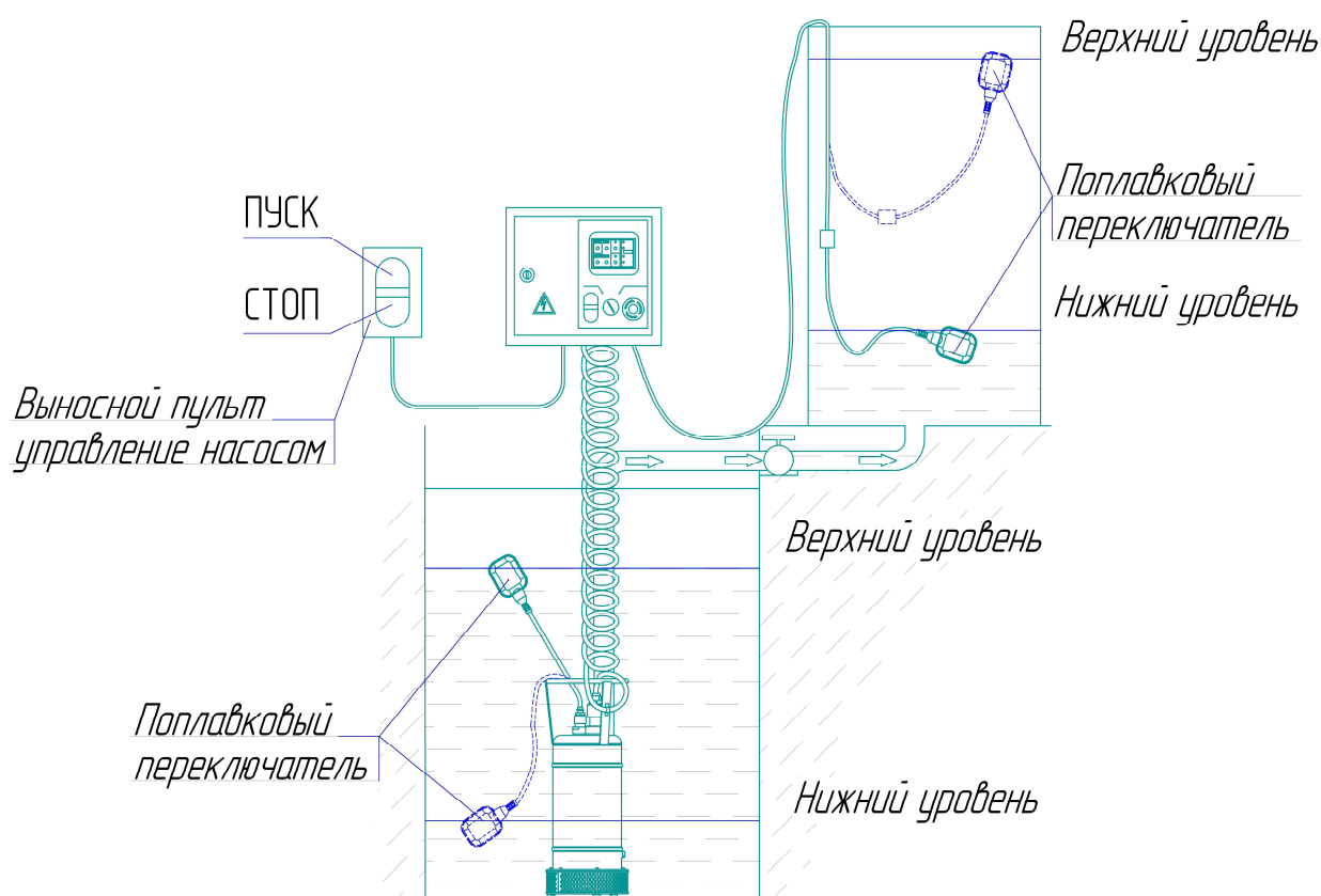
Рисунок Д.3 Пример монтажа станции управления и защиты асинхронного электродвигателя работающего на слив.
