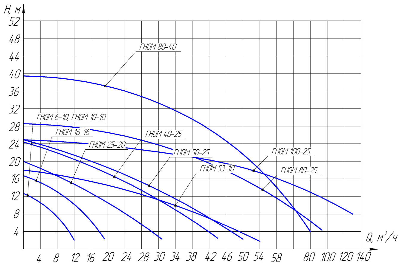
Рисунок Б.1 - Рабочие характеристики электронасосов типа ГНОМ
